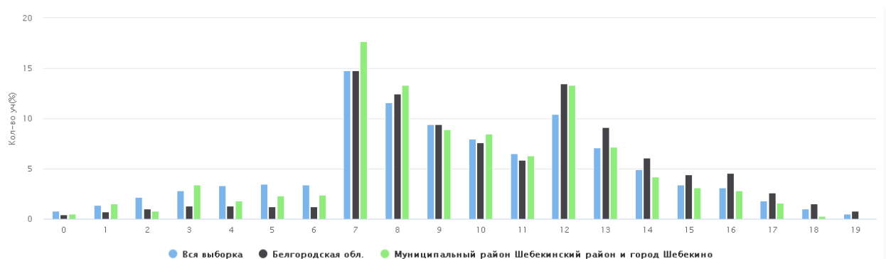
Общая гистограмма первичных баллов ВПР 2020 / 8 Математика
