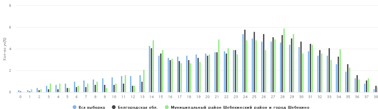
Общая гистограмма первичных баллов ВПР 2020 / 5 Русский язык
