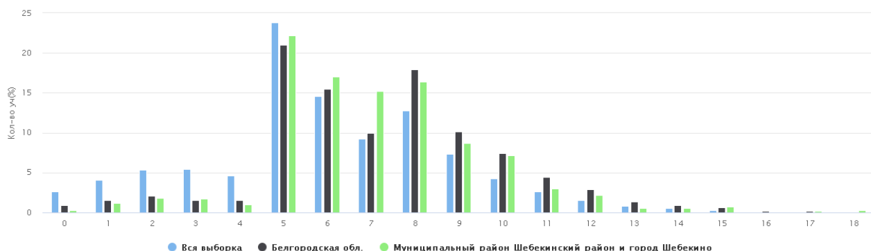
Общая гистограмма первичных баллов ВПР 2020 / 9 Физика
