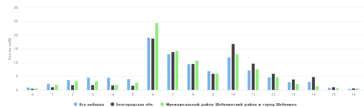
Общая гистограмма первичных баллов ВПР 2020 / 7 Математика
